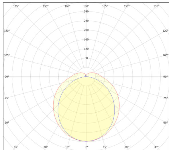
Lichtverteilungskurve
