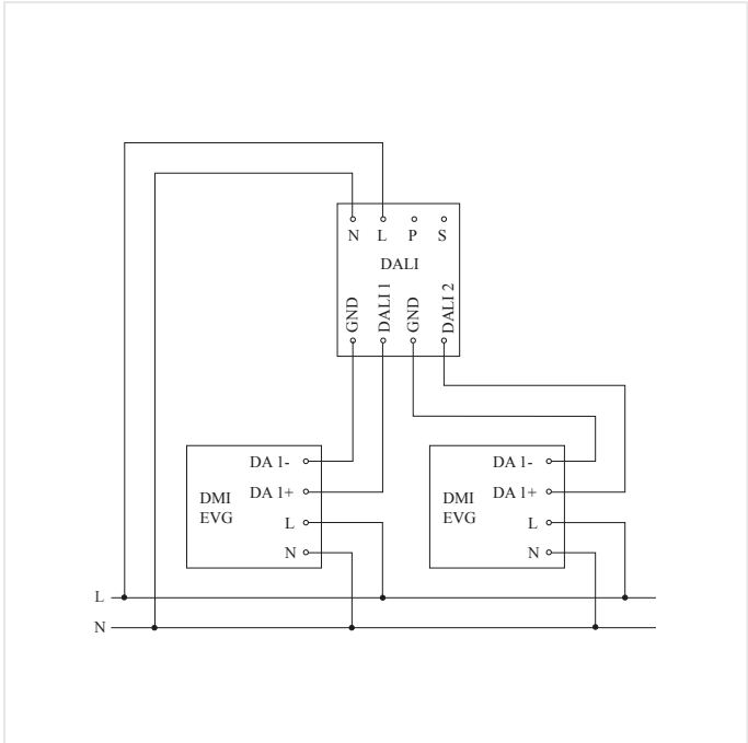
Schaltungsplan Master
