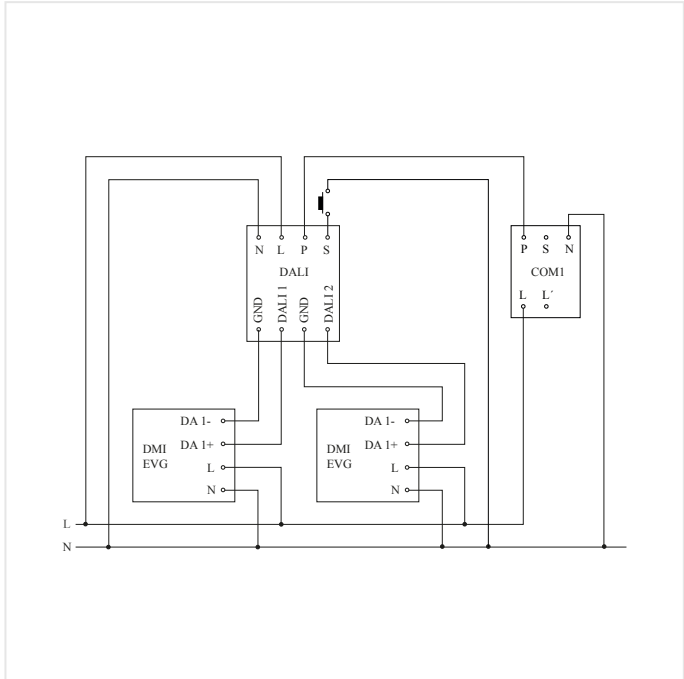
Schaltungsplan Master-Slave Vernetzung
