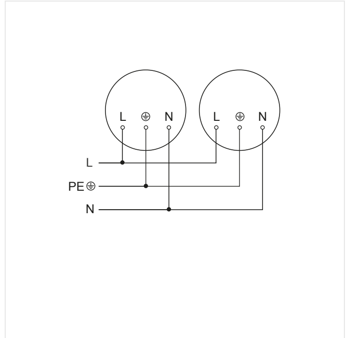
Schaltplan
