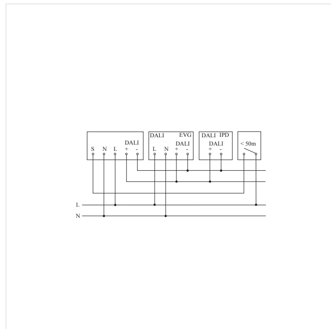
Schéma de câblage pour la mise en réseau DALI-2 APC &amp; DALI-2 IPD
