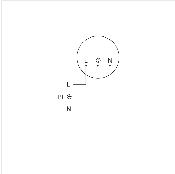
Schaltplan Master
