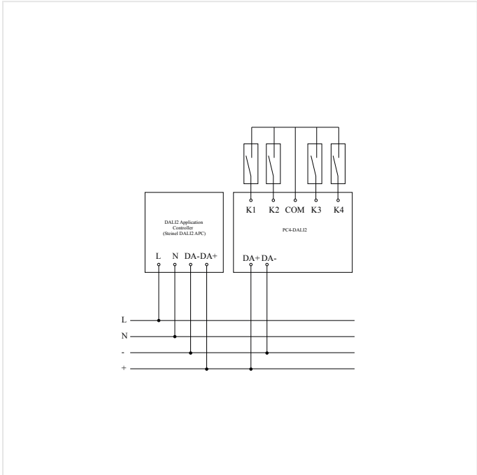
Schaltplan Anschluss 4-fach Tasterkoppler an DALI2 APC
