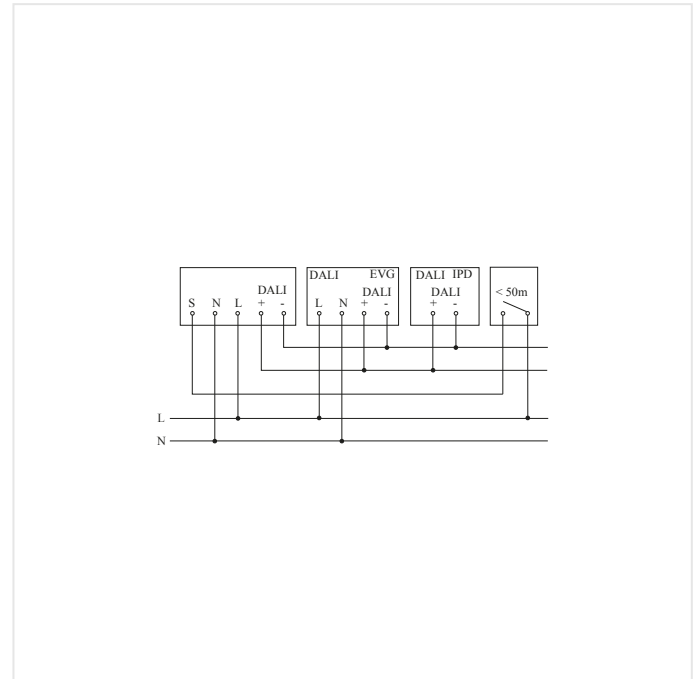
Schéma de câblage pour la mise en réseau DALI-2 APC & DALI-2 IPD
