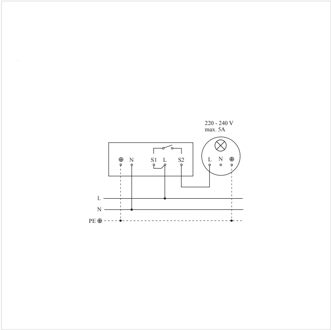
Schéma du circuit principal 230V
