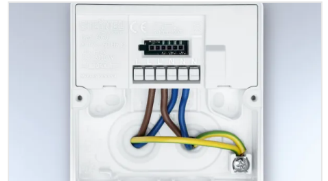
Grande vano per l'allacciamento elettrico
