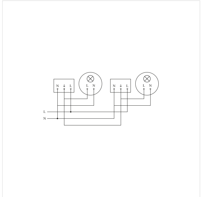
Schéma du circuit d'interconnexion maître/esclave
