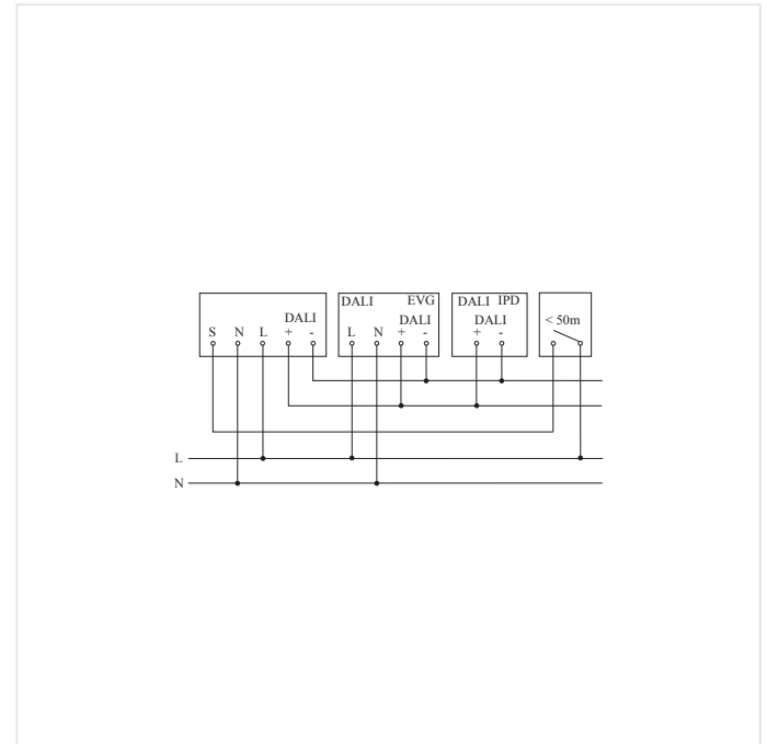
Schema elettrico collegamento in rete di DALI-2 APC & DALI-2 IPD
