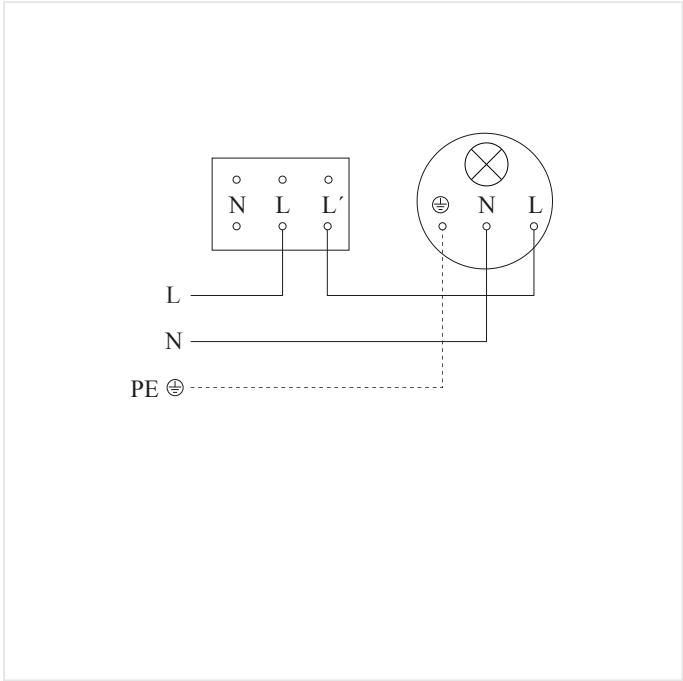
Schaltplan 2-Draht-Verkabelung
