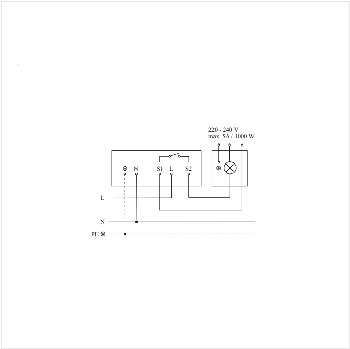
Schema elettrico Master PF
