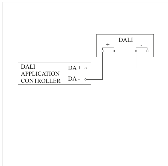
Schema elettrico collegamento in rete di DALI-2 APC &amp; DALI-2 IPD
