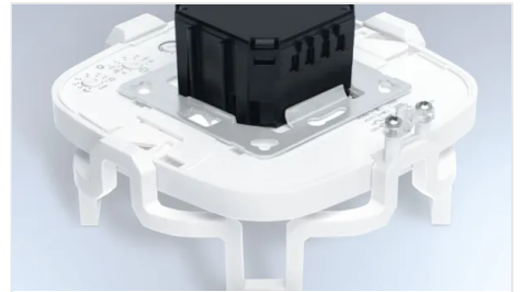
HF Deckenadapter zur Montage auf abgehängten Decken
