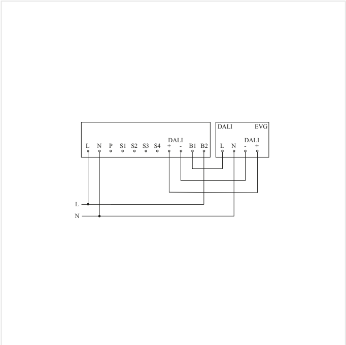
Schaltplan Master mit EVG aus
