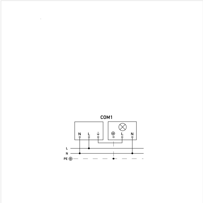
Schaltplan 3-Draht-Verkabelung
