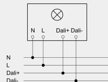
Schaltbild DALI Wiring diagram DALI Schéma de circuit DALI Schema elettrico DALI
