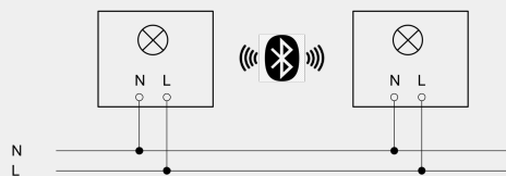
Schaltbild Connect Wiring diagram Connect Schéma de circuit Connect Schema elettrico Connect
